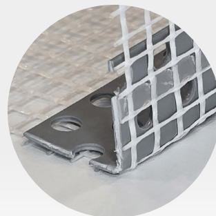
Rete incollata tramite una singola striscia di colla per una maggiore resistenza. PPLARETE25-02
