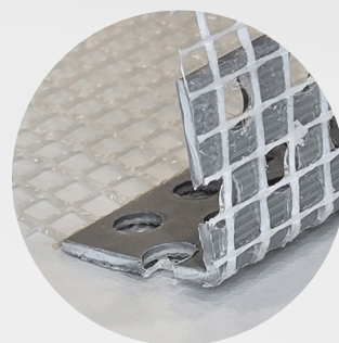
Rete incollata su tutta la lunghezza del profilo. PPLARETE25-01
