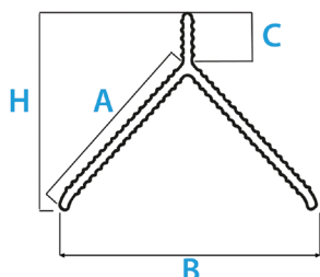
Paraspigolo a Lama
