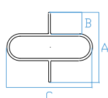
DISTANZIATORE PIATTO
